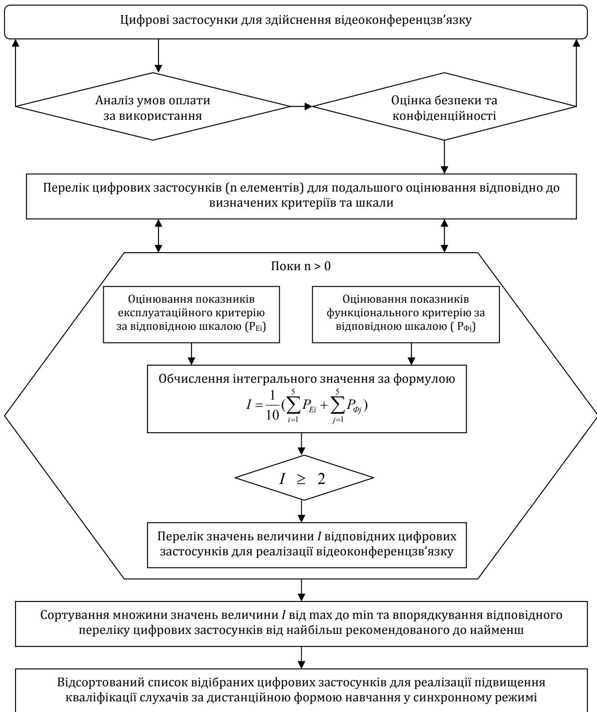
Рис. Блок-схема алгоритму вибору цифрового застосунку для реалізації підвищення кваліфікації за дистанційною формою навчання у синхронному режимі
